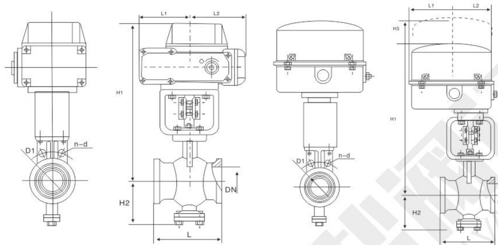
电子式内伺服ZDJV-16型 Electronic servo ZDJV-16 type within
