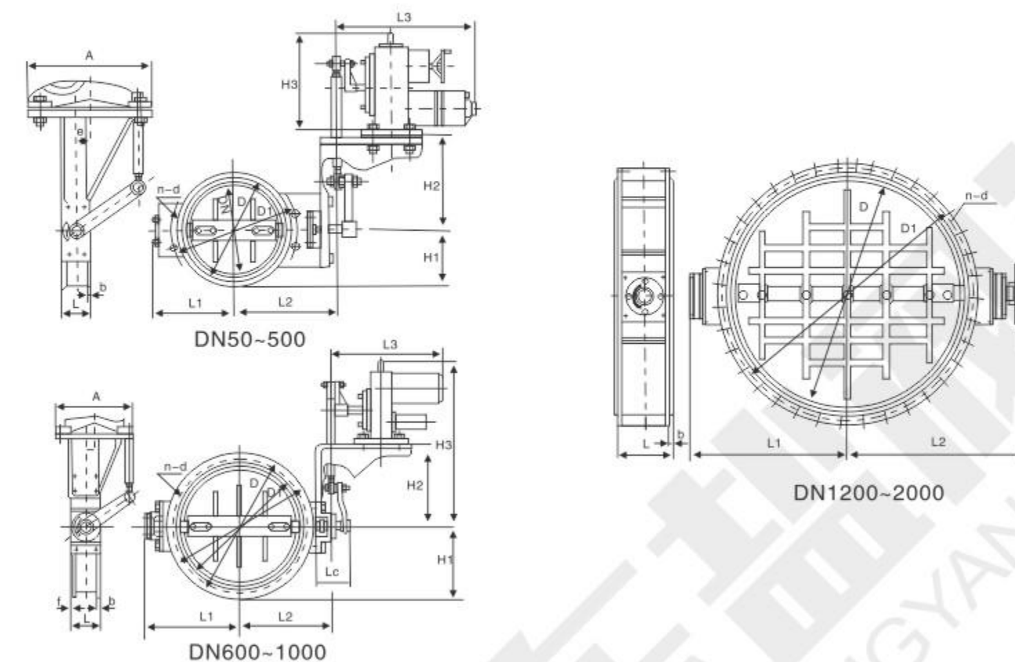
外形尺寸External dimension
