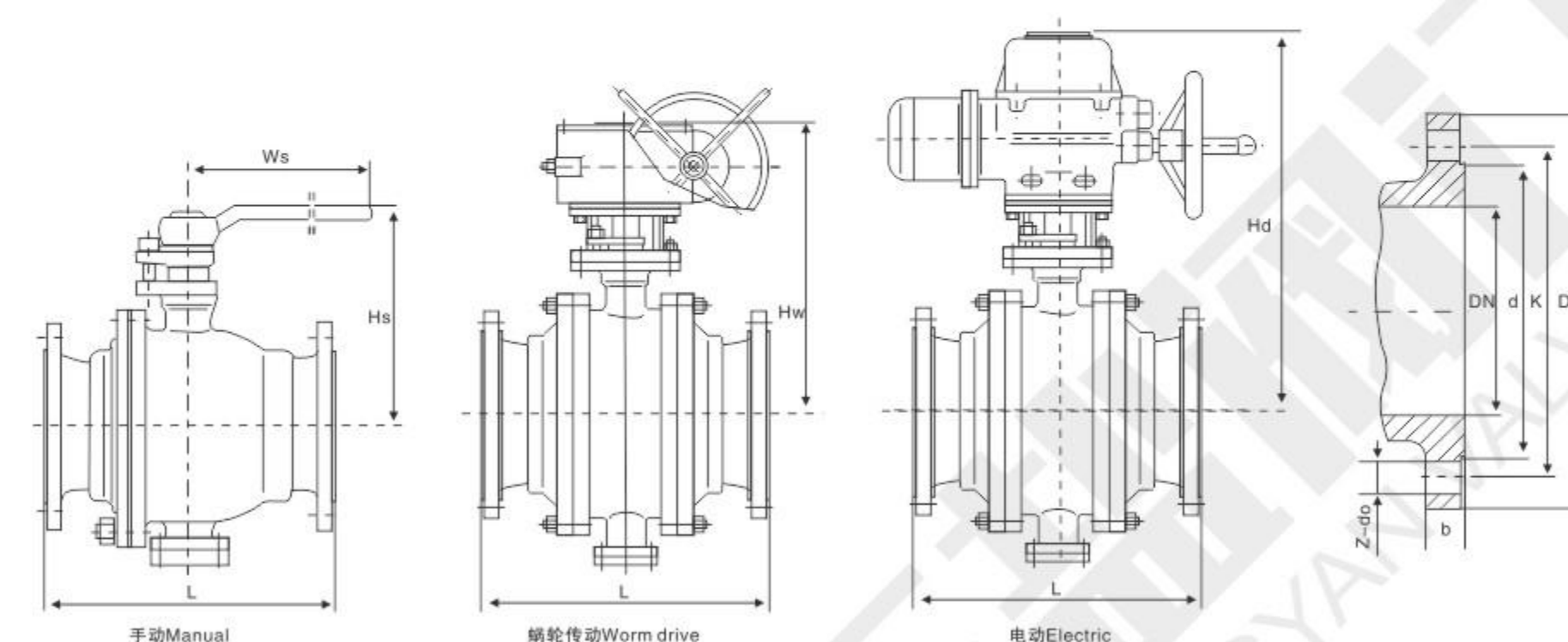
主要连接尺寸Main connection dimensions
